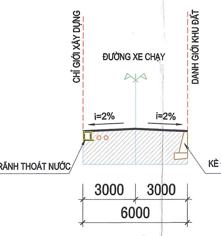
MẶT CẮT 2-2 TỶ LỆ 1/250
