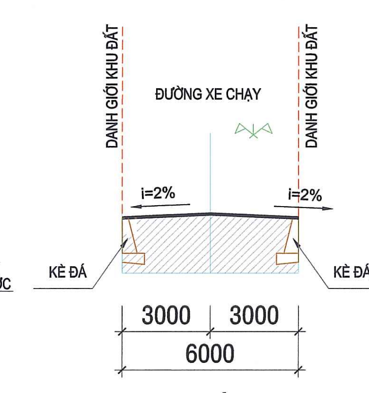
MẶT CẮT 4-4 TỶ LỆ 1/250
