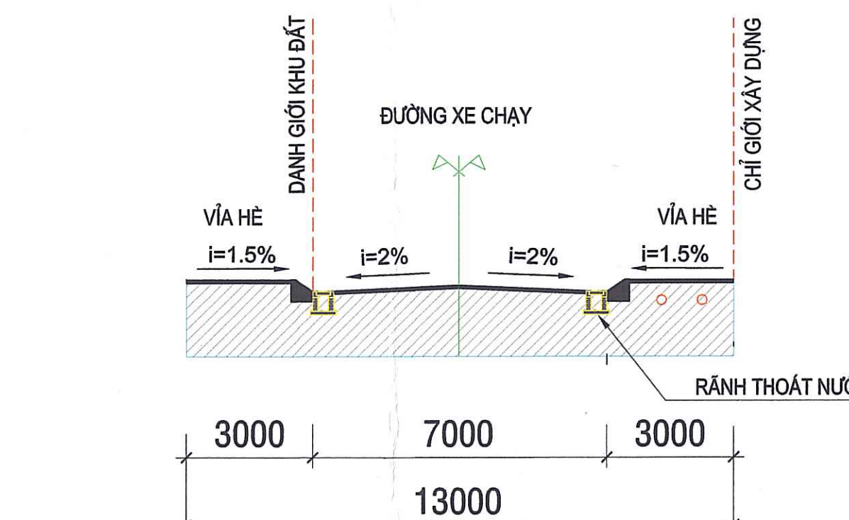
MẶT CẮT 1-1 TỶ LỆ 1/250
