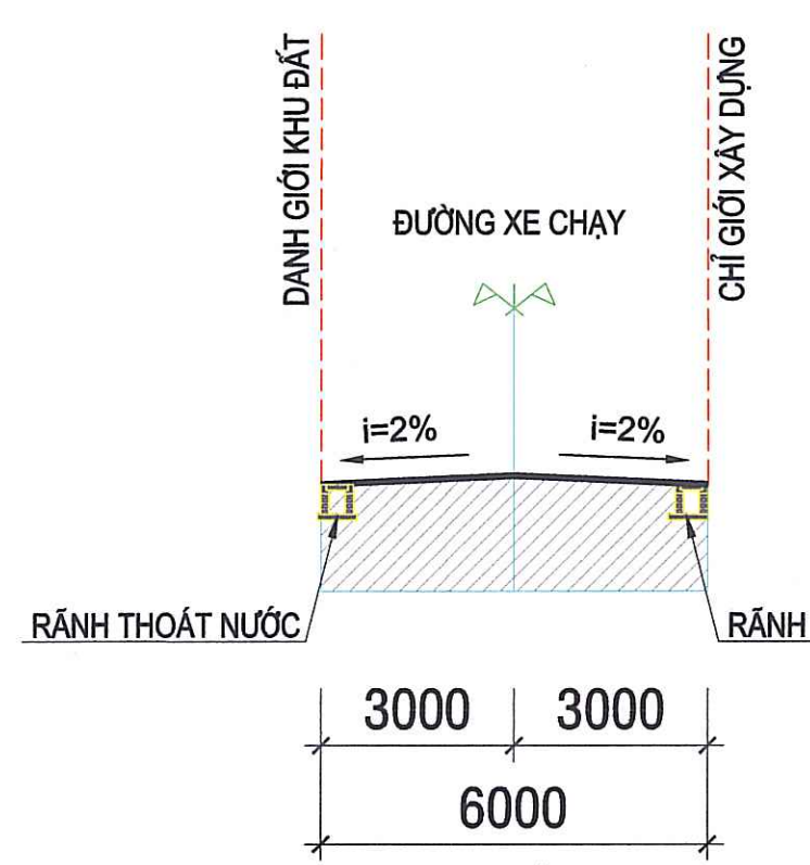
MẶT CẮT 3-3 TỶ LỆ 1/250
