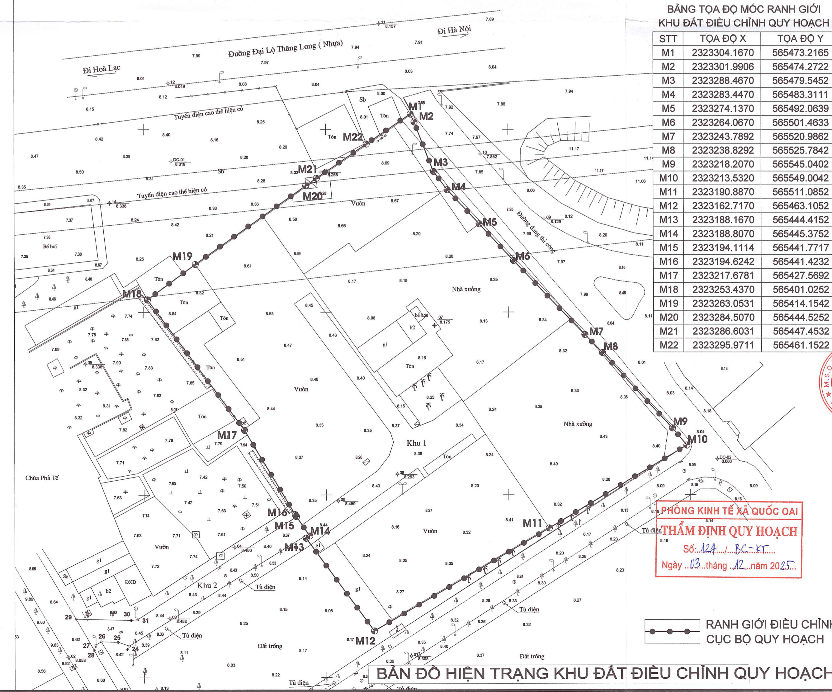
VỊ TRÍ KHU ĐẤT ĐIỀU CHỈNH CỤC BỘ QUY HOẠCH (X) TRONG DỰ ÁN KHU NHÀ Ở CAO CẤP NGÔI NHÀ MỚI
