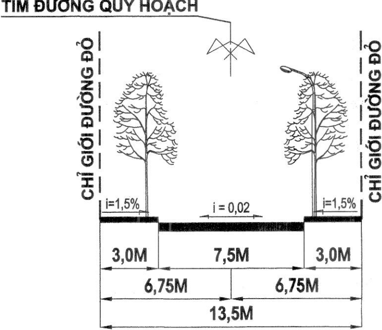
MẶT CẮT NGANG ĐIỂN HÌNH, TỶ LỆ 1/200
